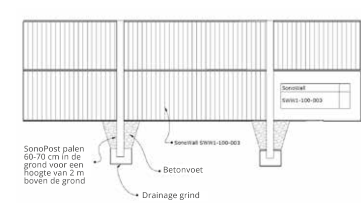
Voorbeeld configuratie op 2 m hoogte met SonoPost houten palen
